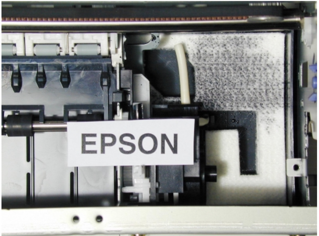
Abbildung 3 : Drucker mit Epson-Tinte, Fliess unter der Ansaugereinrichtung
