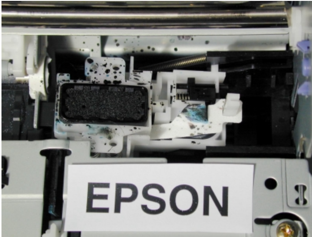
Abbildung 1 : Absaugereinrichtung des Druckers mit Epson-Tinte
